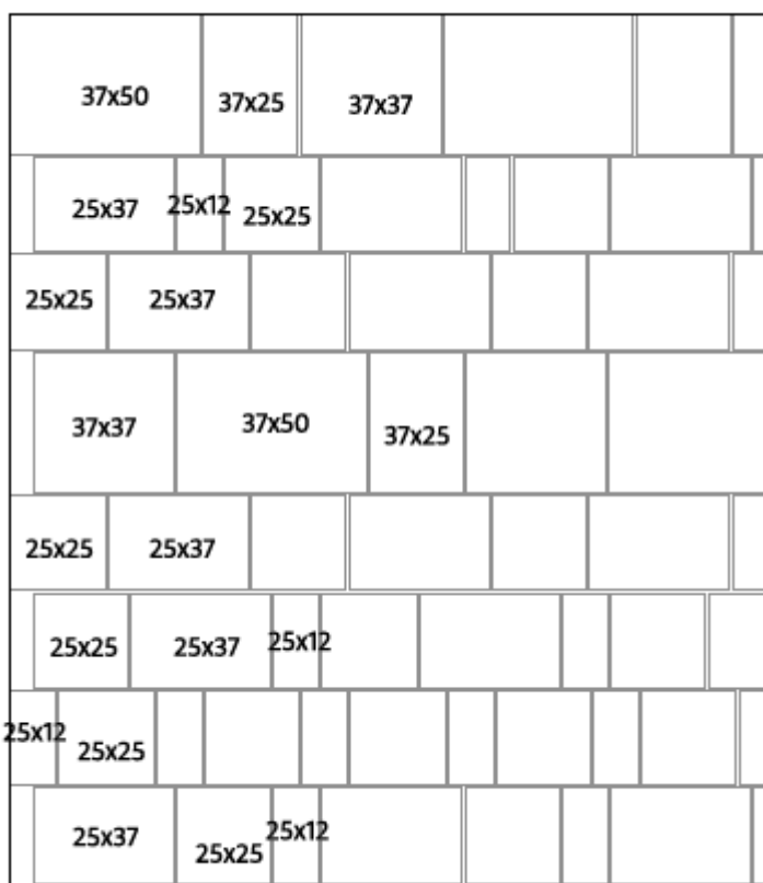
DETALL PATRÓ 1:25
